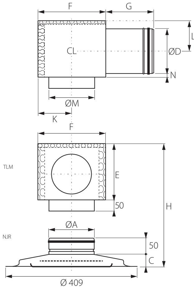
Billede 4. Målskitse (mm), loftdiffuser NJR og trykfordelingsboks TLM.
